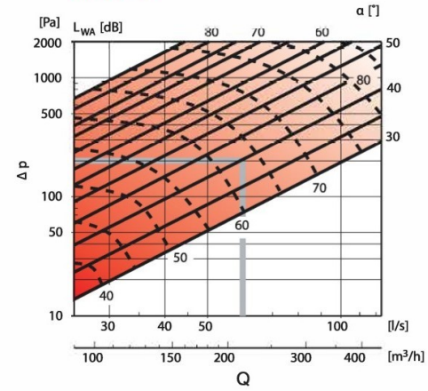
AKH Ø160
