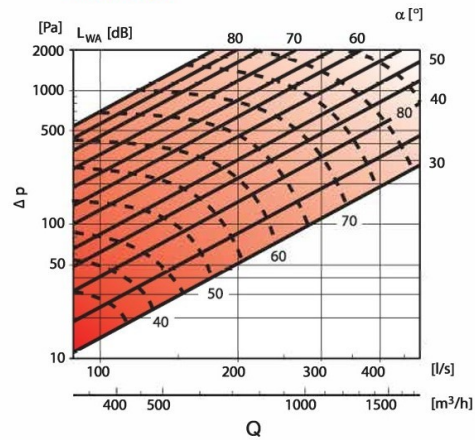
AKH Ø200
