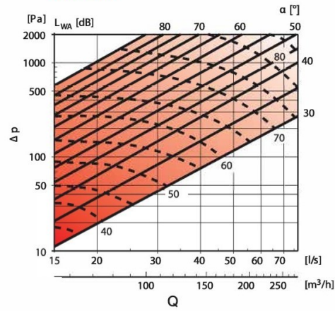
AKH Ø125
