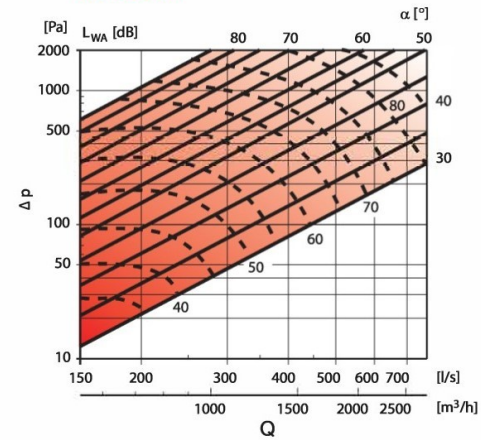
AKH Ø250
